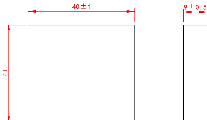
4. 变压器顶部导热垫尺寸 (受限于机箱高度, 导热垫厚度可相应调整)
