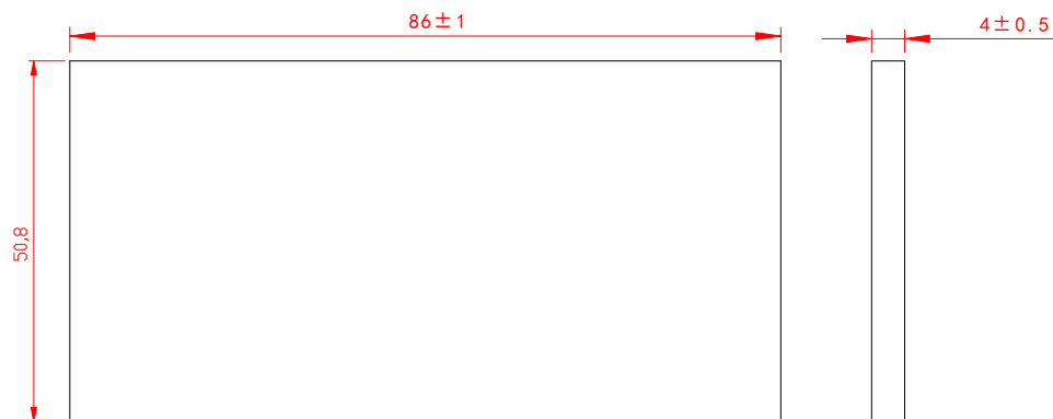
5. 电源底部导热垫尺寸 (受限于机箱铆柱高度, 导热垫厚度可相应调整)
