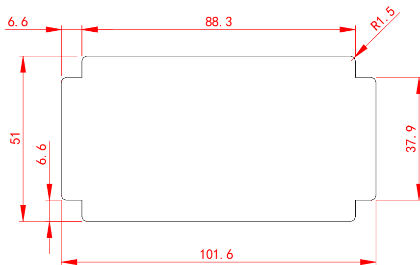
6. 电源底部麦拉片尺寸 (厚度 0.25 \pm 0.05\text{mm} )
